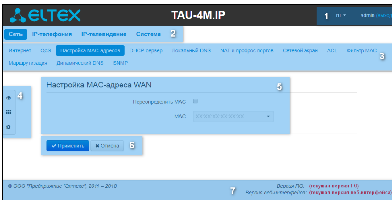
Рисунок 7 – Элементы навигации Web-конфигуратора
