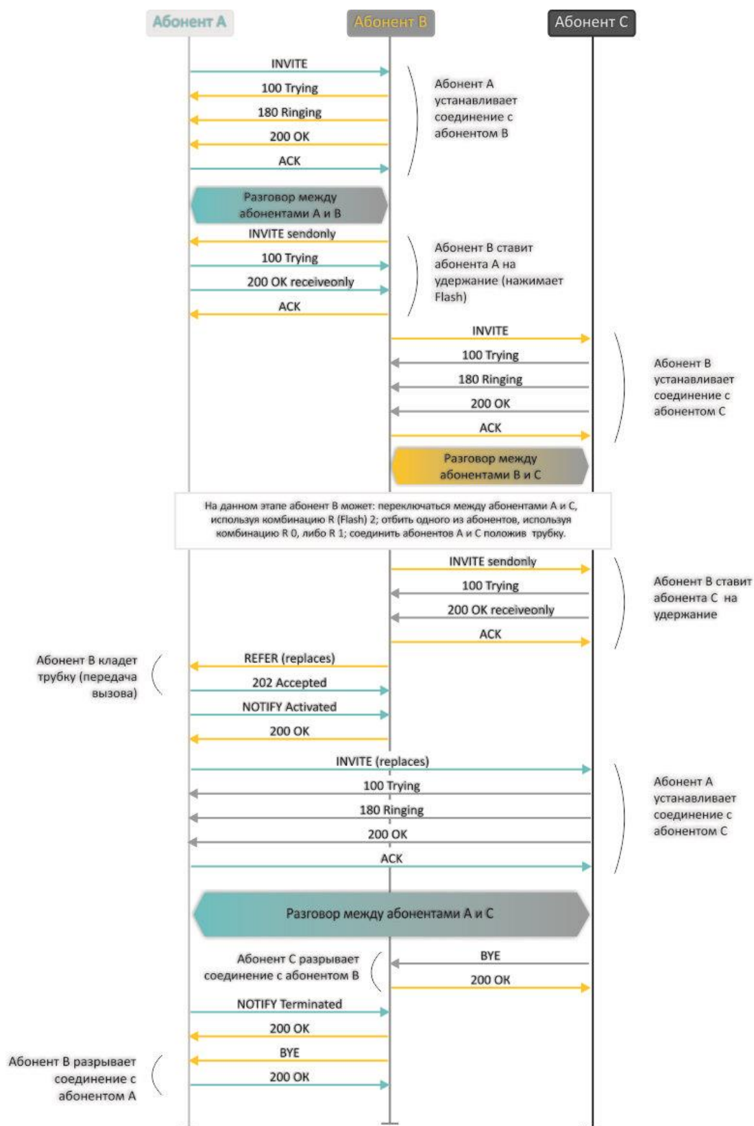
Рисунок 16 – Алгоритм выполнения услуги «Сопровождаемый перевод вызова» («Attended calltransfer») абонентом «В» по протоколу SIP
