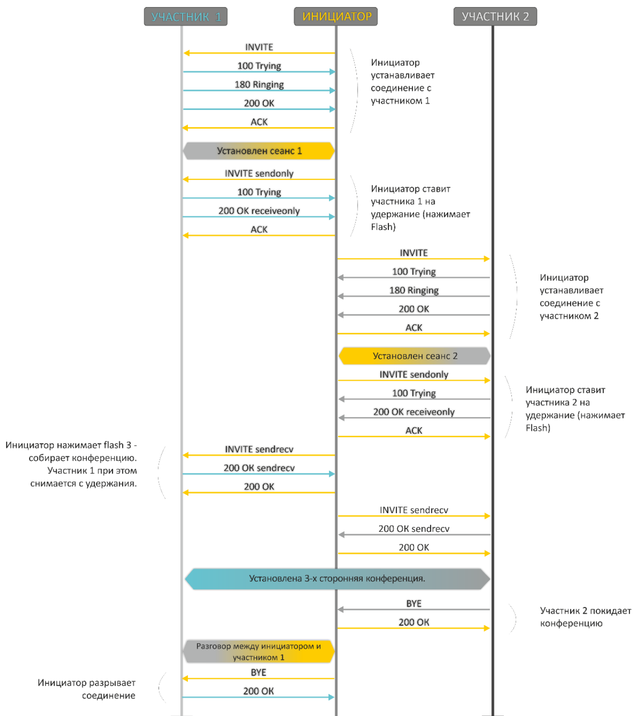
Рисунок 18 – Алгоритм выполнения услуги «Трёхсторонняя конференция» («3-way conference») локально на устройстве по протоколу SIP
