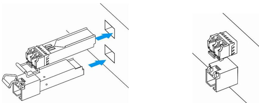
Рисунок 14 – Установка SFP-трансиверов
