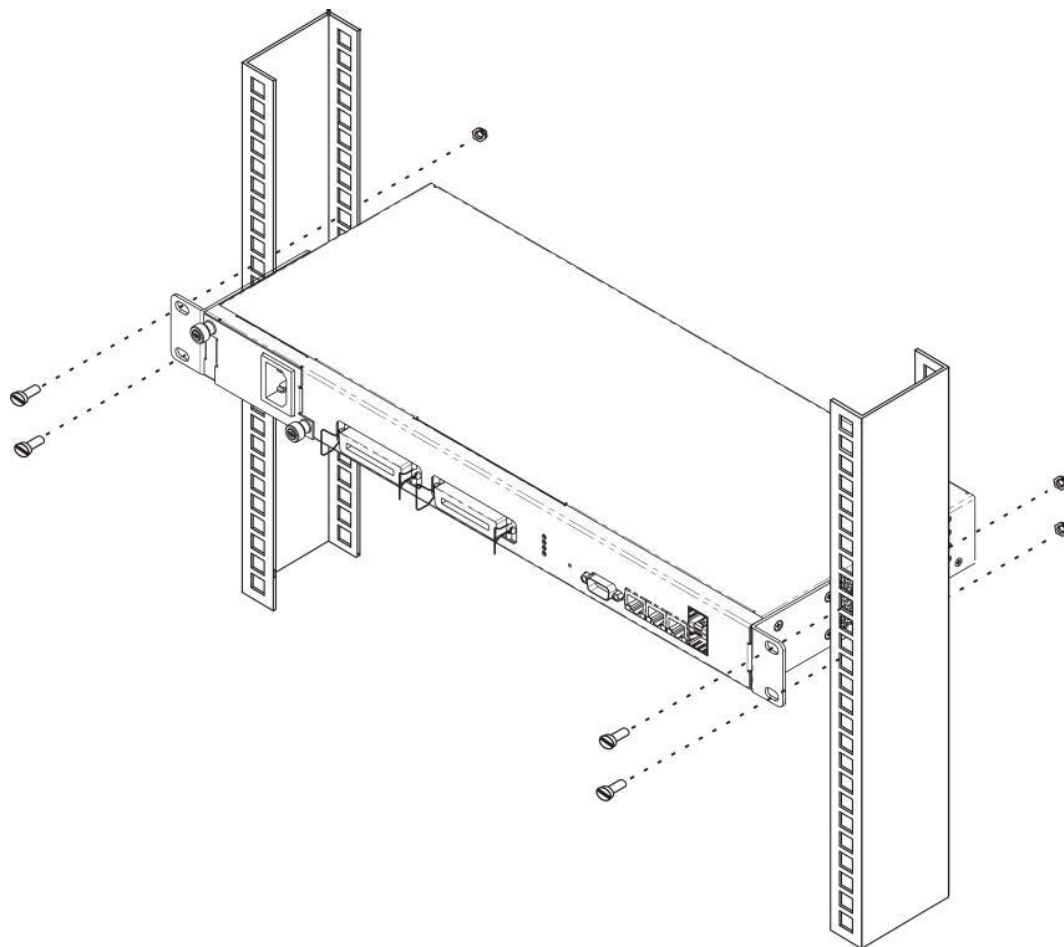
Рисунок 11 – Установка устройства в стойку
