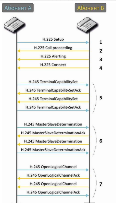
Рисунок 24 – Алгоритм вызова по протоколу H.323
