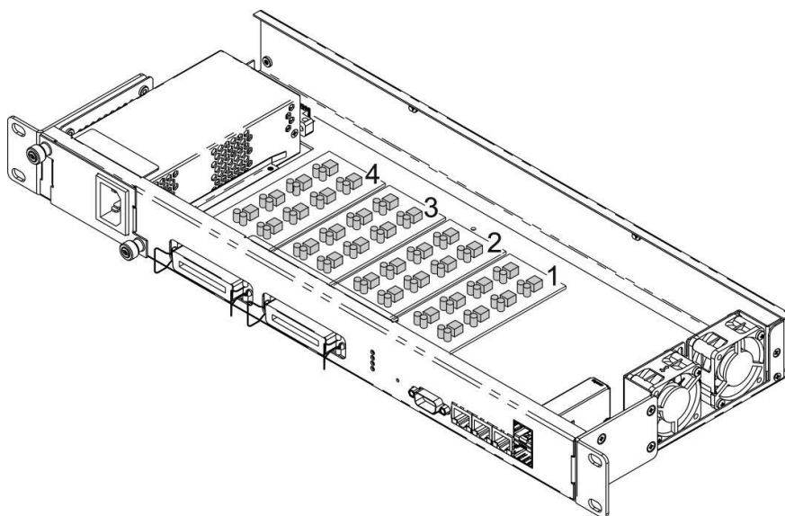
Рисунок 13 – Расположение субмодулей в TAU-32M.IP
