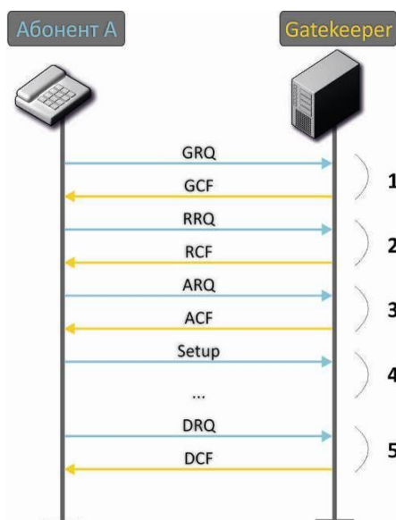
Рисунок 25 – Алгоритм вызова через гейткипер
