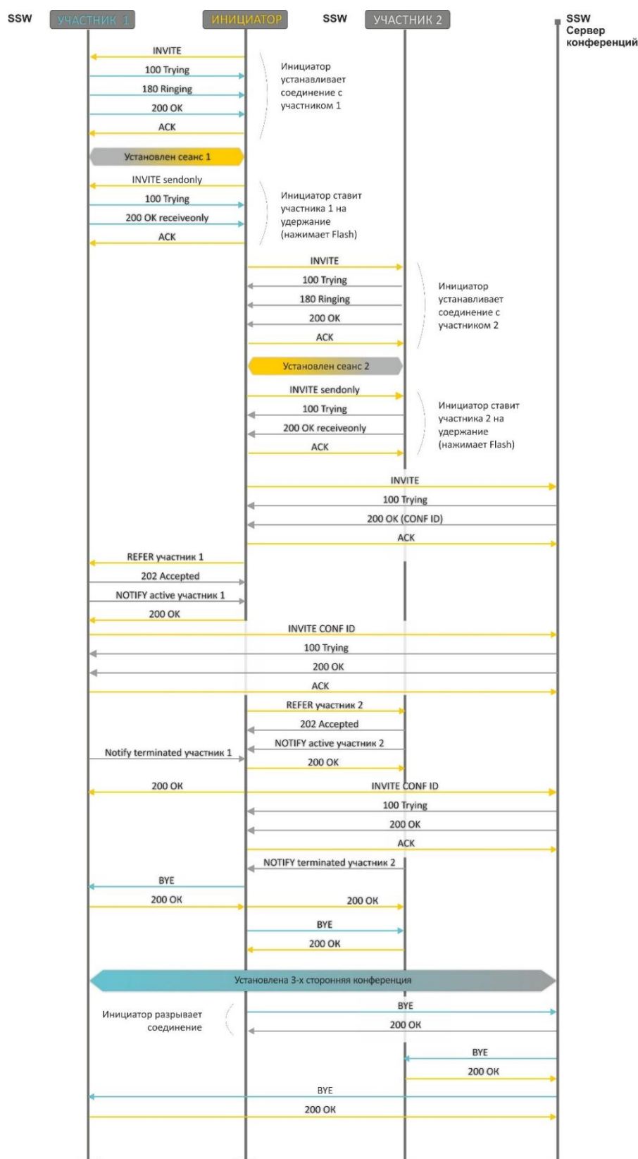
Рисунок 20 – Алгоритм выполнения услуги «Трёхсторонняя конференция» («3-way conference») на сервере конференций по протоколу SIP (REFER to user)
