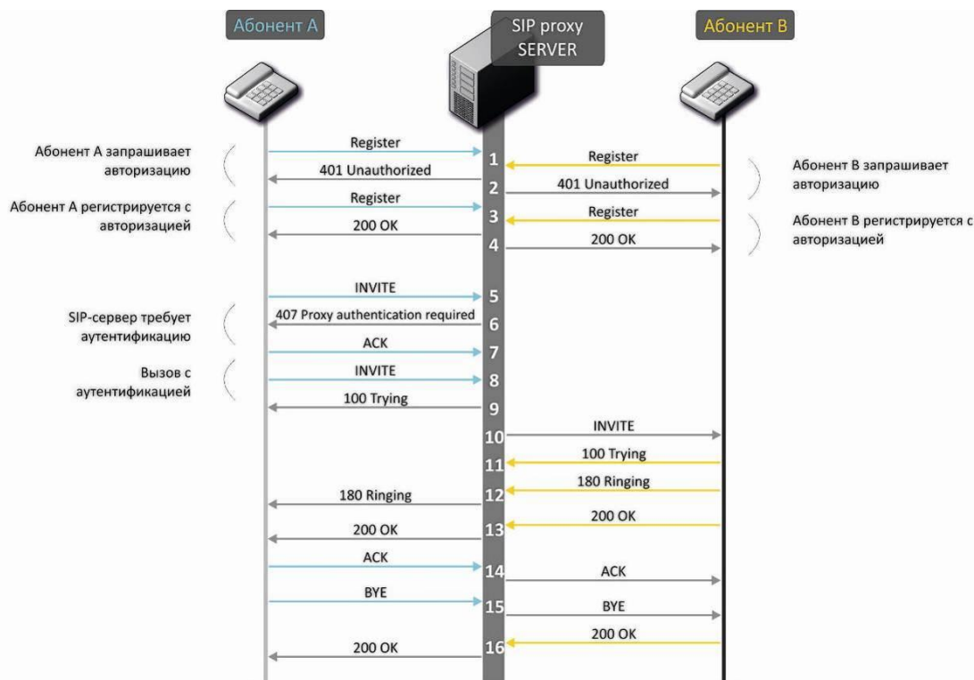
Рисунок 22 – Алгоритм вызова с участием SIP проху-сервера
