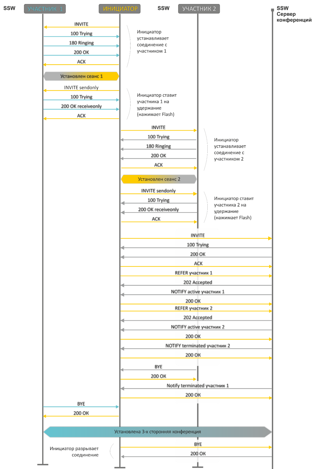
Рисунок 19 – Алгоритм выполнения услуги «Трёхсторонняя конференция» («3-way conference») на сервере конференций по протоколу SIP (REFER to focus)
