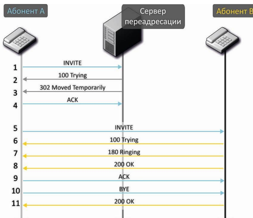
Рисунок 23 – Алгоритм вызова с участием сервера переадресации
