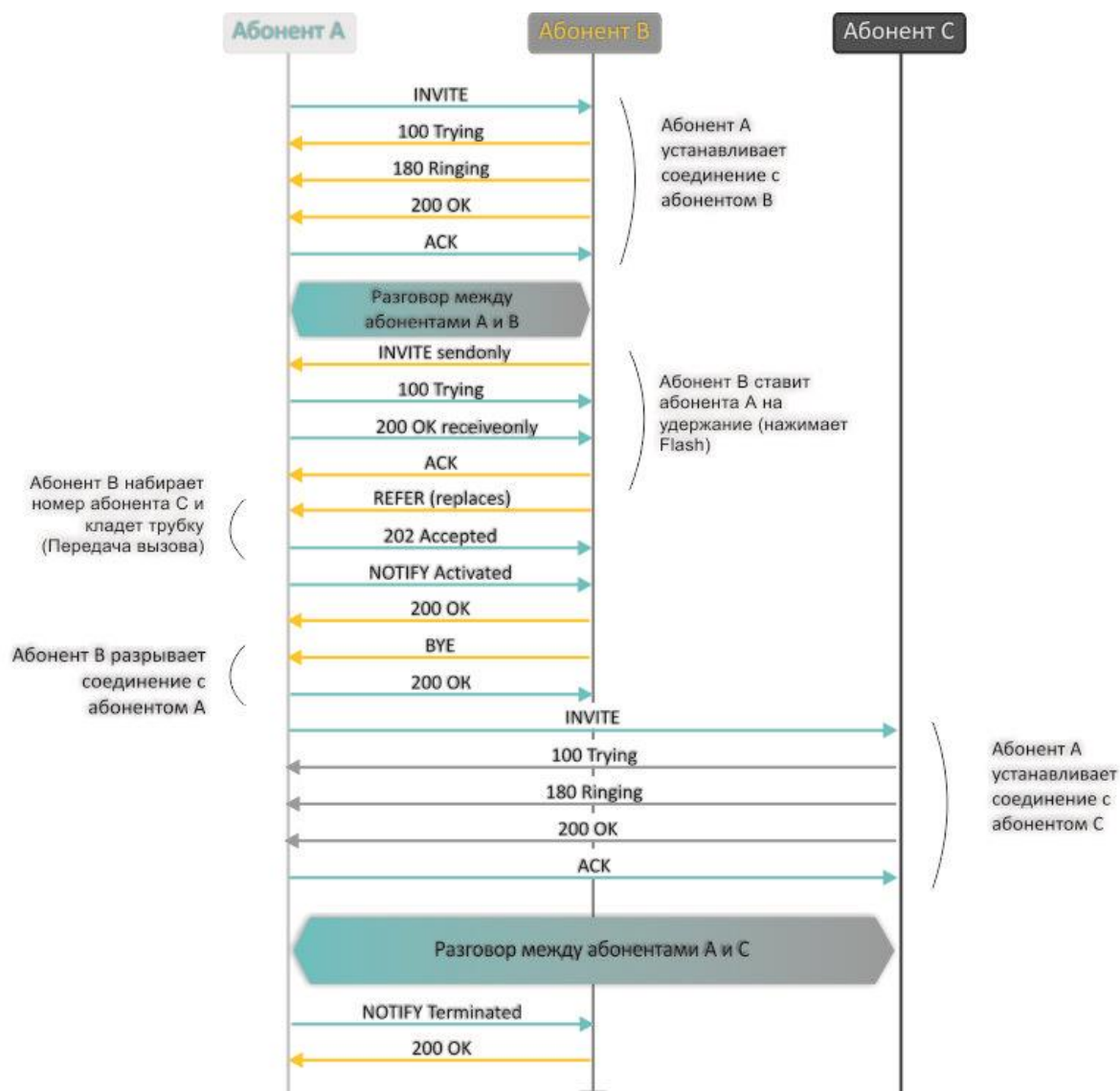
Рисунок 17 – Алгоритм выполнения услуги «Перевод вызова без сопровождения» («Unattended calltransfer») абонентом «В» по протоколу SIP
