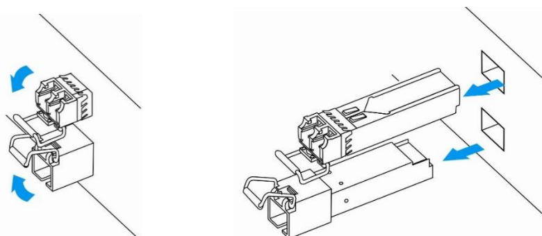
Рисунок 15 – Открытие защелки SFP-трансиверов и извлечение SFP-трансиверов
