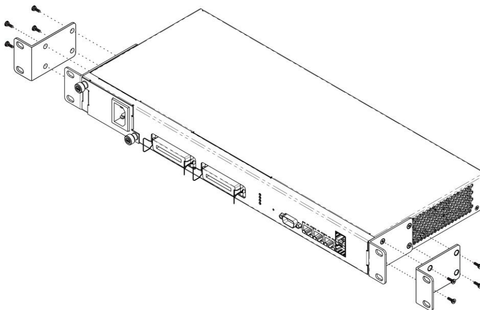
Рисунок 10 – Крепление кронштейнов
