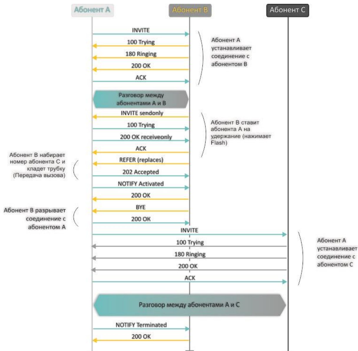
Рисунок 9 – Алгоритм выполнения услуги «Перевод вызова без сопровождения» («Unattended calltransfer») абонентом В по протоколу SIP
