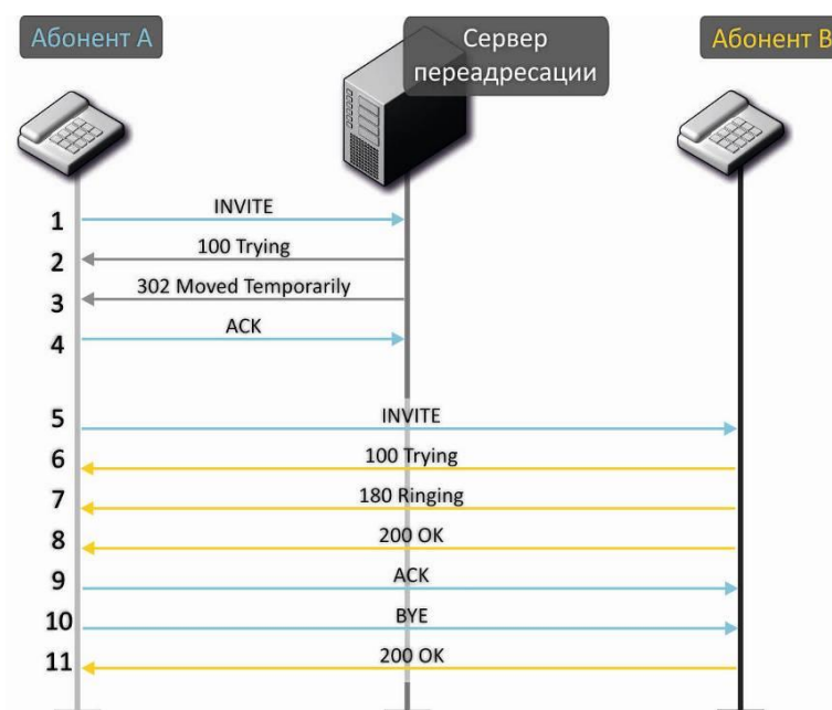
Рисунок 16 – Алгоритм вызова с участием сервера переадресации
