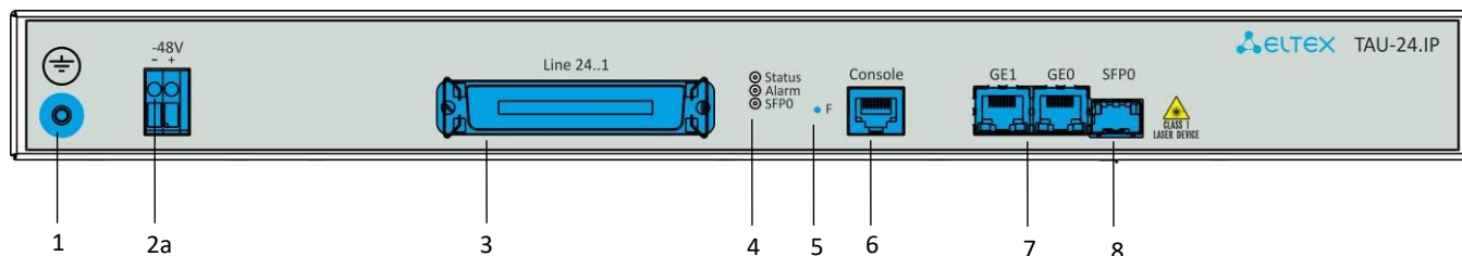
Рисунок 4в – Внешний вид передней панели TAU-24.IP с питанием от постоянного тока
