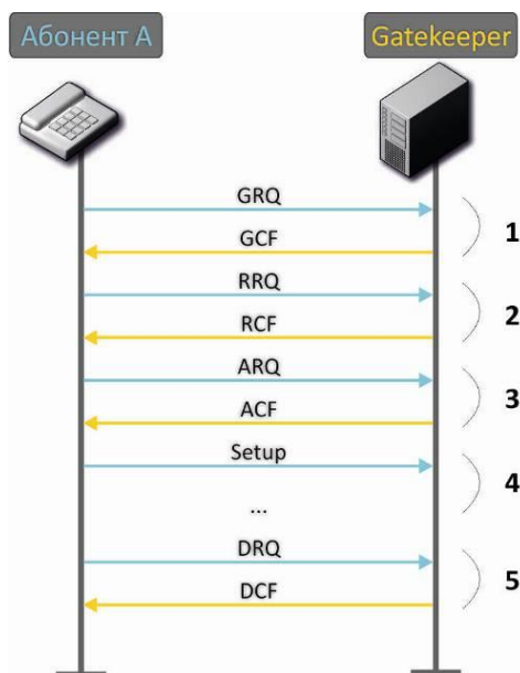
Рисунок 18 – Алгоритм вызова через гейткипер
