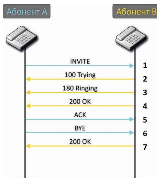
Рисунок 14 – Алгоритм вызова по протоколу SIP
