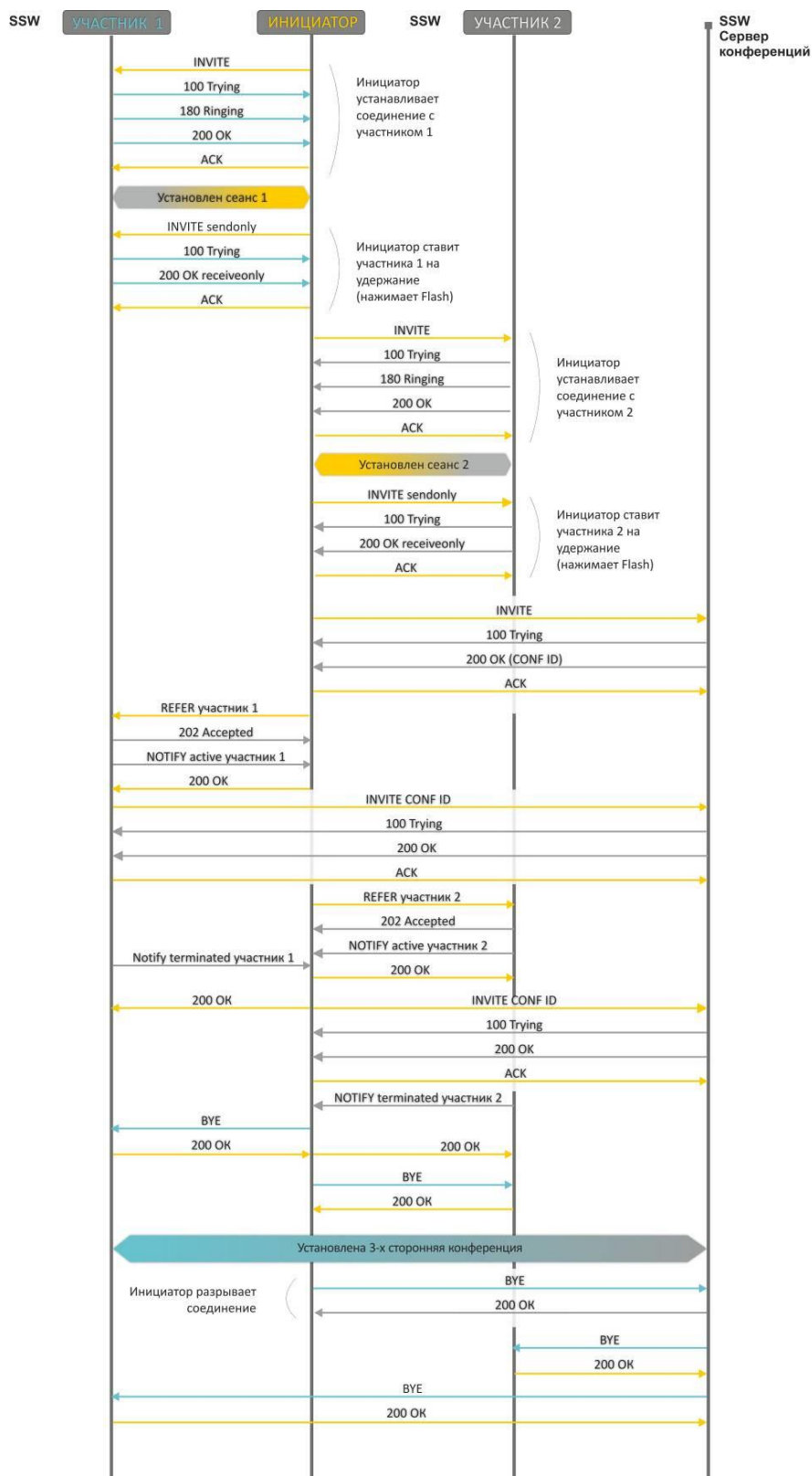
Рисунок 13 – Алгоритм выполнения услуги «Трёхсторонняя конференция» («3-way conference») на сервере конференций по протоколу SIP (REFER to user)
