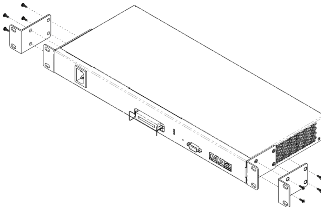
Рисунок 6 – Крепление кронштейнов
