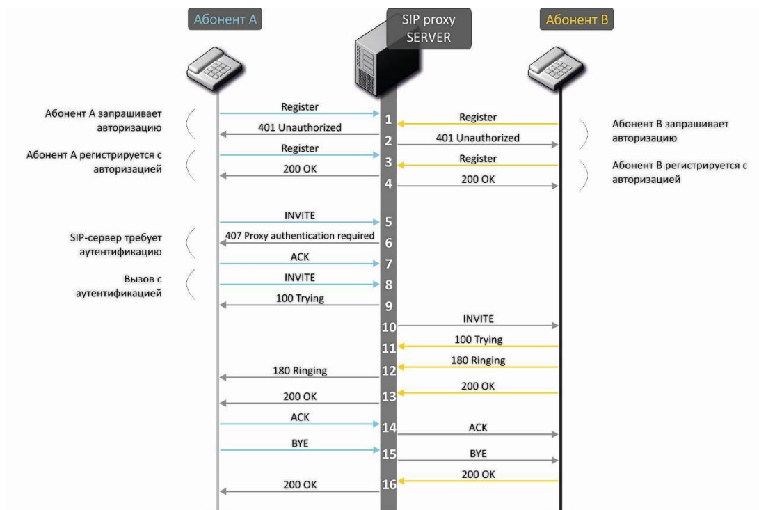
Рисунок 15 – Алгоритм вызова с участием SIP проху-сервера
