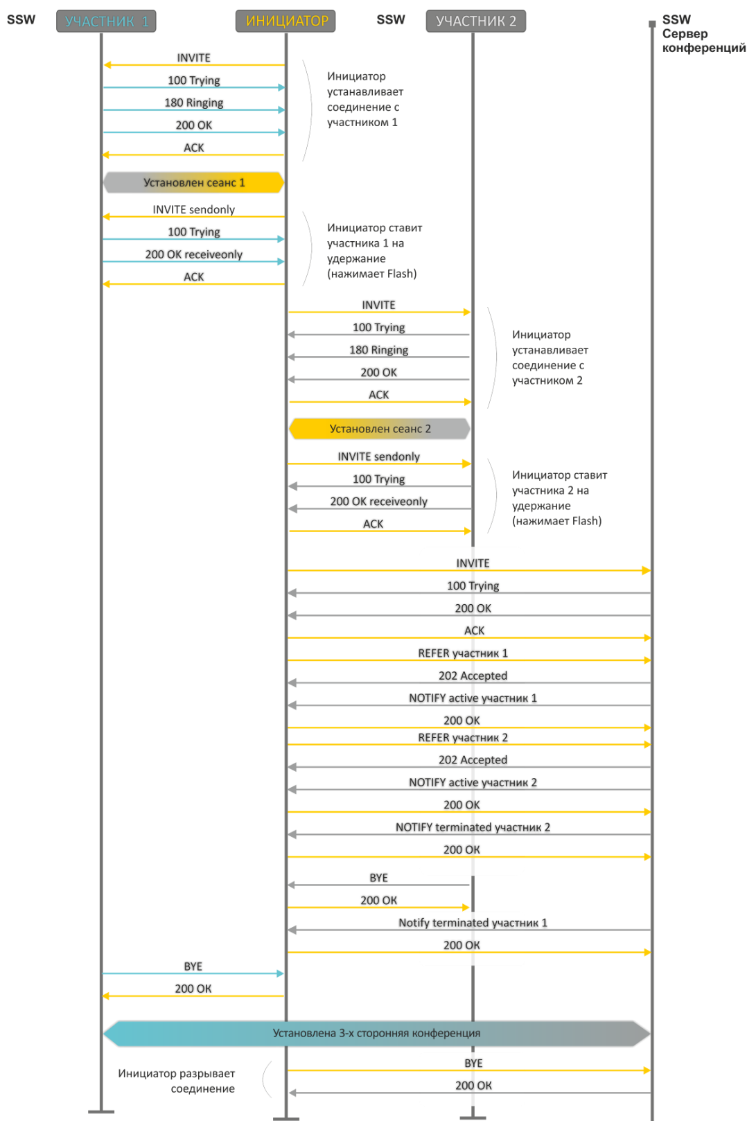
Рисунок 12 – Алгоритм выполнения услуги «Трёхсторонняя конференция» («3-way conference») на сервере конференций по протоколу SIP (REFER to focus)
