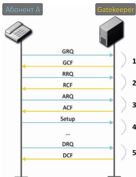
Рисунок 18 – Алгоритм вызова через гейткипер
