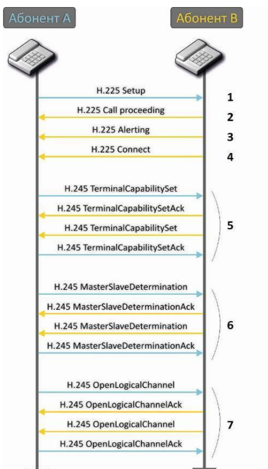
Рисунок 17 – Алгоритм вызова по протоколу H.323
