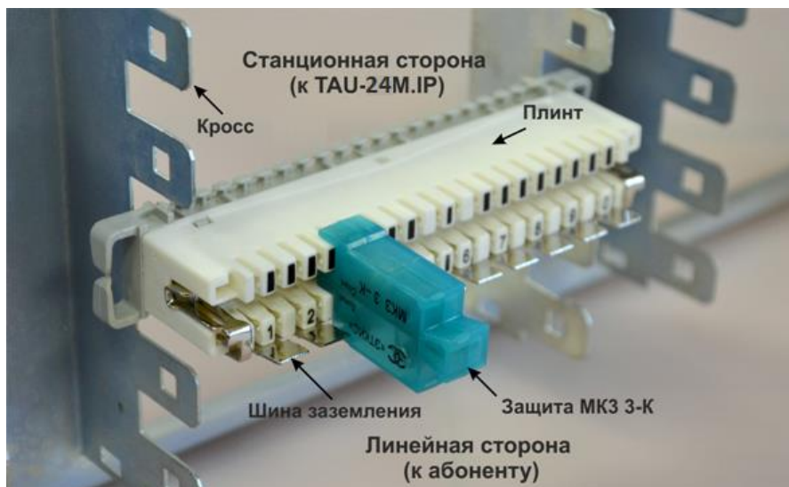
Рисунок 5 – Схема подключения
