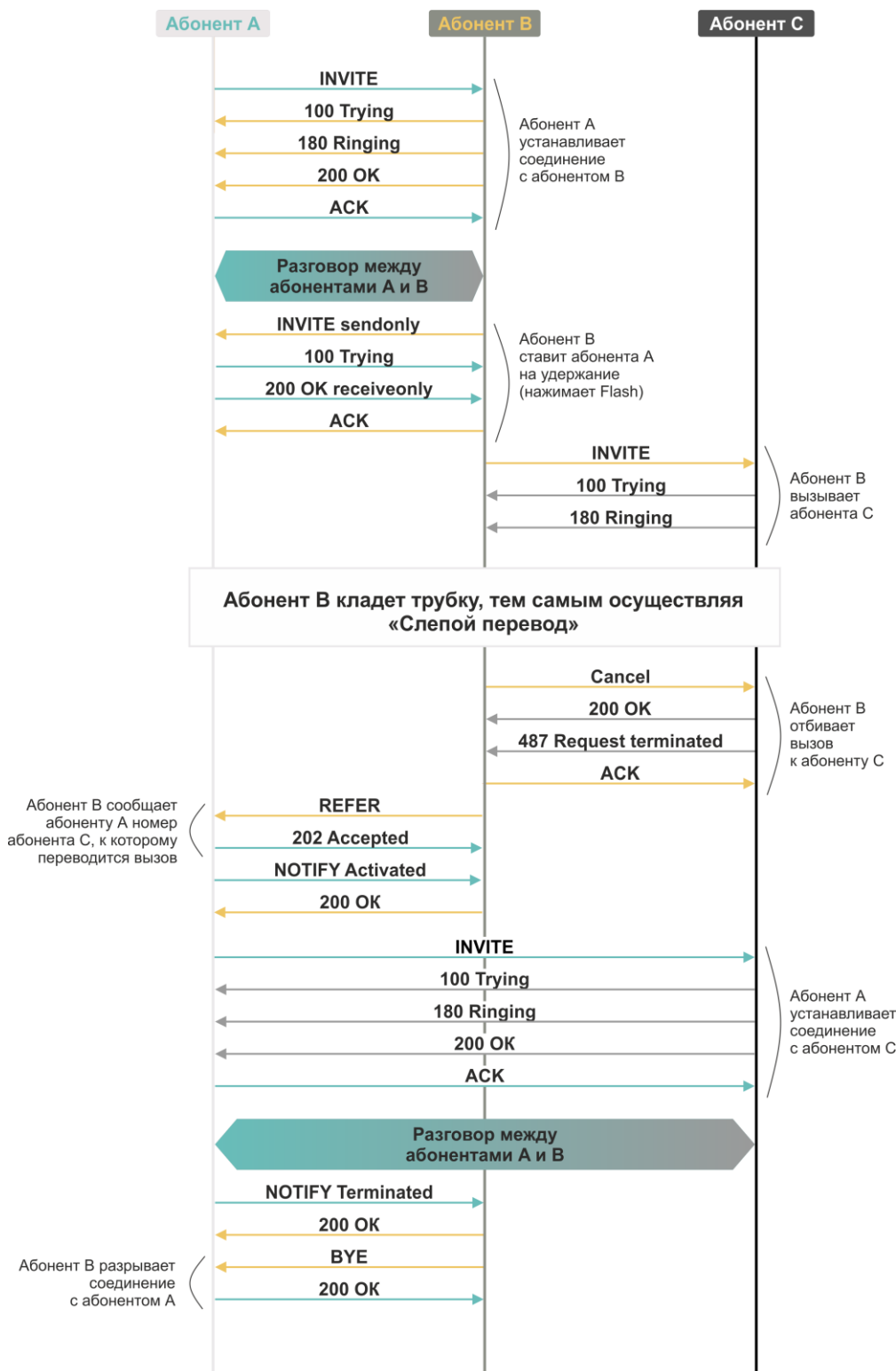
Рисунок 10 – Алгоритм выполнения услуги « Blind attended transfer » абонентом В по протоколу SIP
