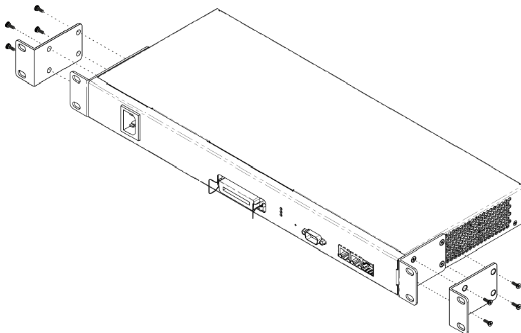
Рисунок 6 – Крепление кронштейнов
