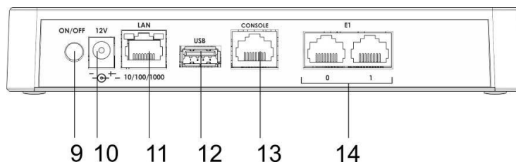
Рисунок 8б – Внешний вид SMG-2. Задняя панель
