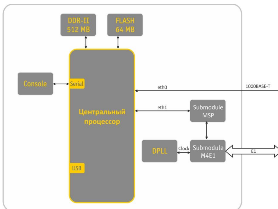
Рисунок 5 – Функциональная схема SMG
