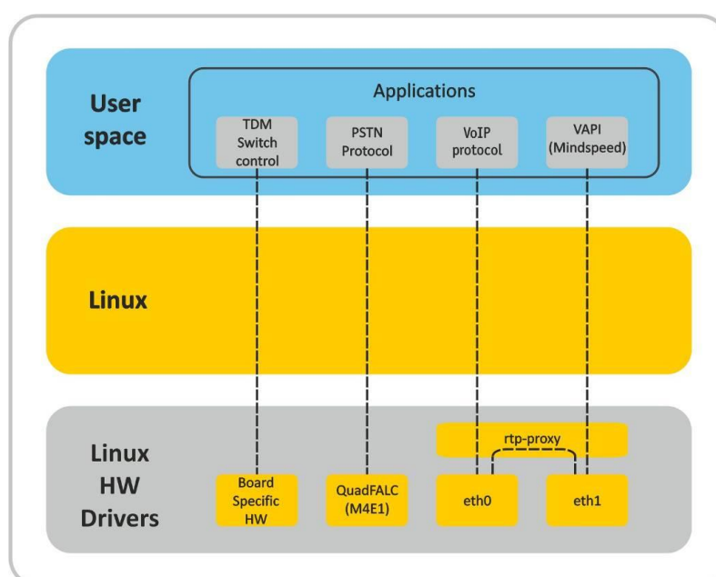
Рисунок 6 – Структура программного обеспечения SMG
