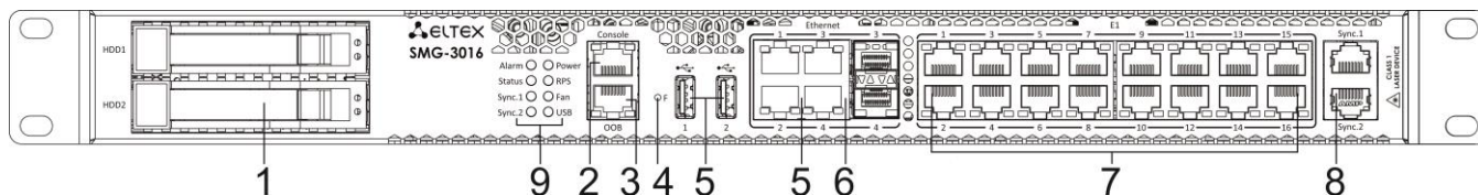
Рисунок 8 — Внешний вид передней панели SBC-3000 (на базе SMG-3016)
