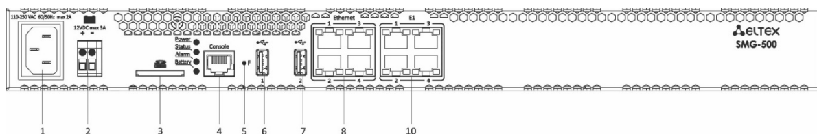
Рисунок 7 — Внешний вид передней панели SMG-500
