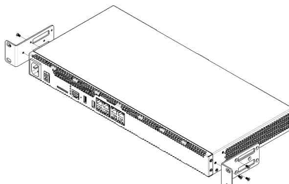
Рисунок 9 — Крепление кронштейнов
