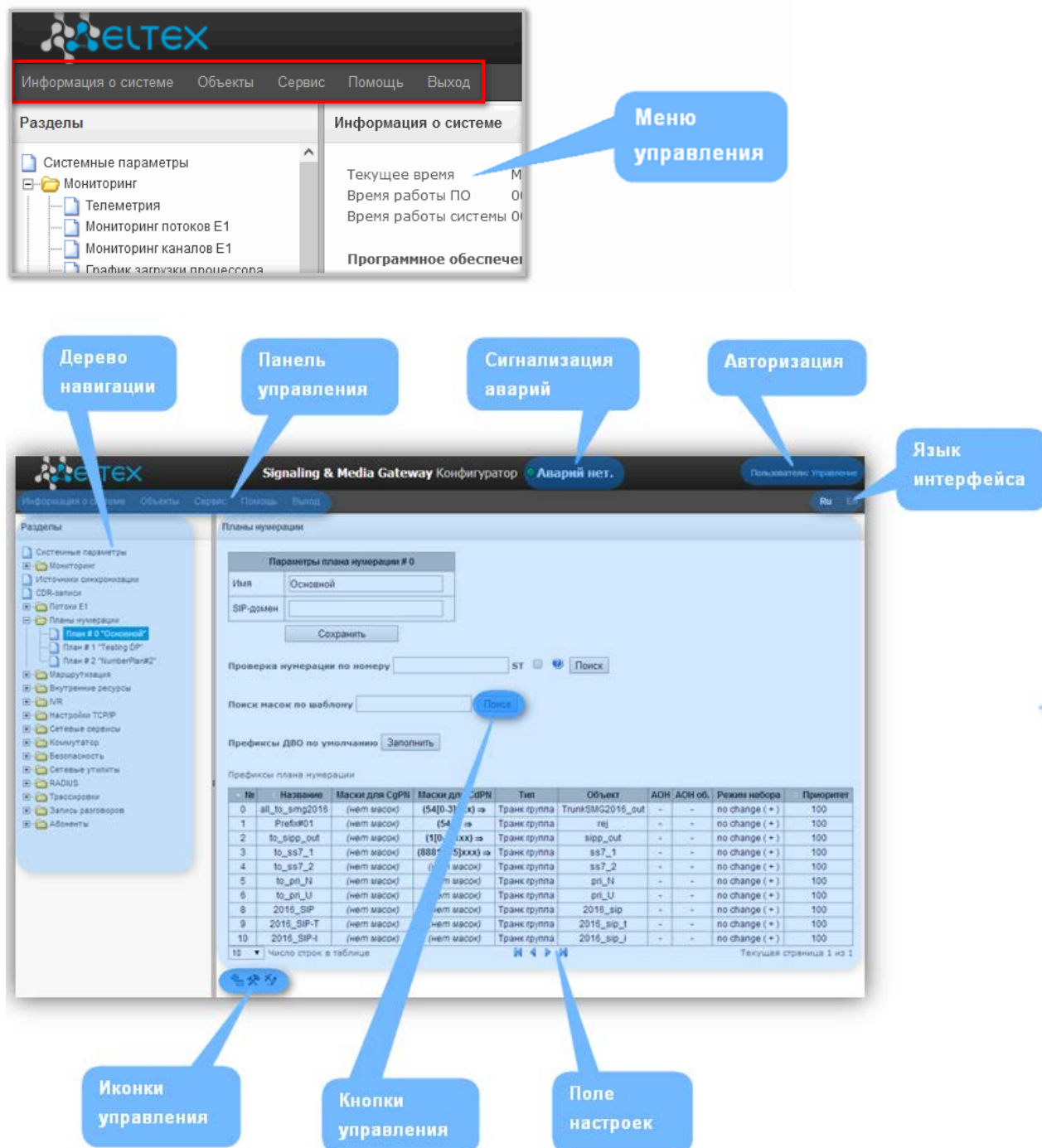
Рисунок 16 — Элементы навигации web-конфигуратора
