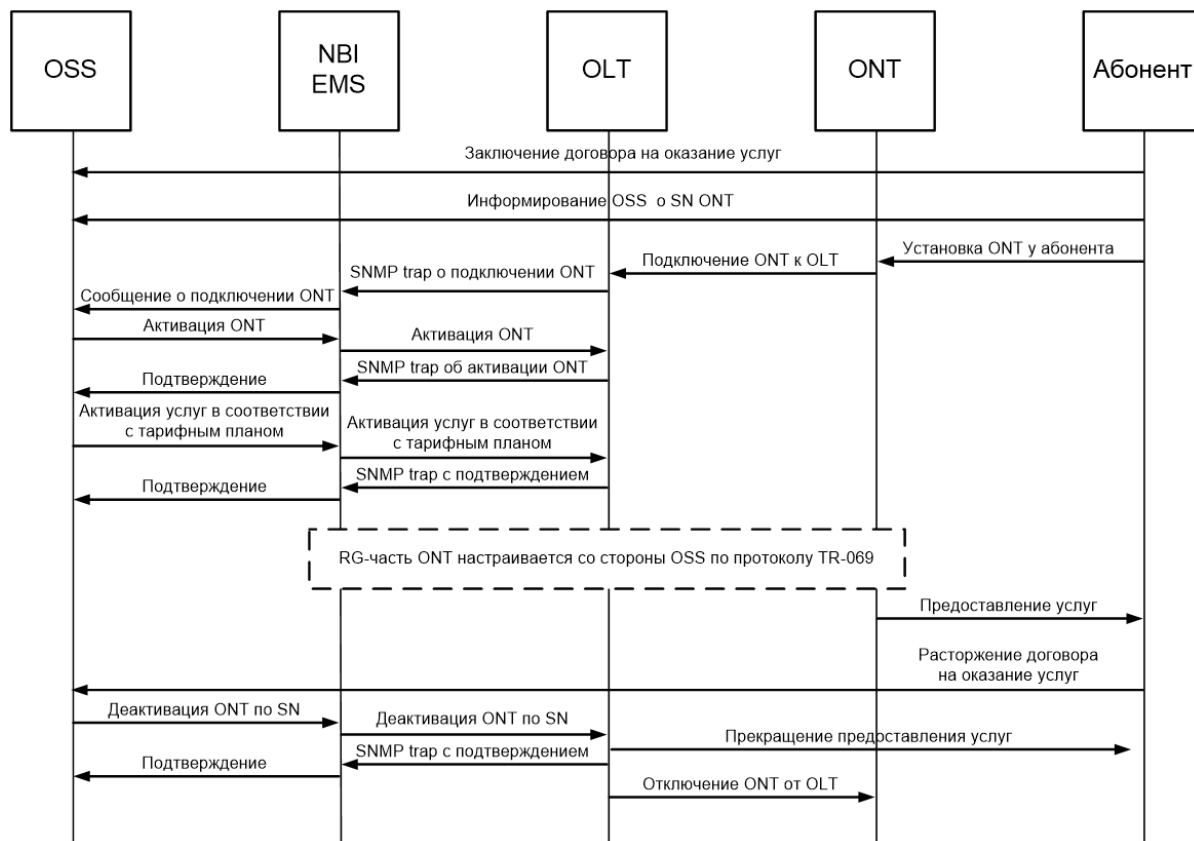
Рисунок 26 – Схема обмена сообщениями между OSS и ONT при активации ONT после установки абоненту
