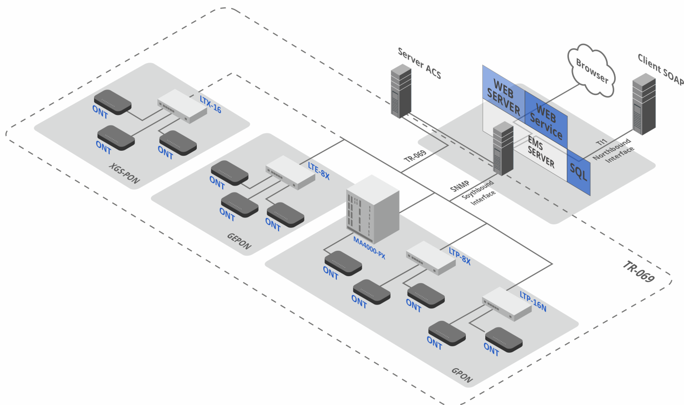
Рисунок 1 – Структура системы управления «Eltex.EMS» для сети с коммутацией и маршрутизацией пакетов информации
