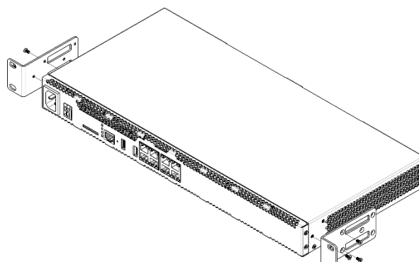
Рисунок 9 — Крепление кронштейнов
