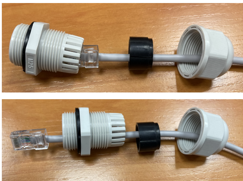
Рисунок 19 — Установка корпуса кабельного ввода на кабеле
