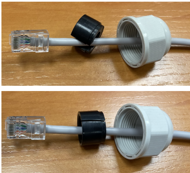
Рисунок 18 — Установка резиновой втулки на кабеле
