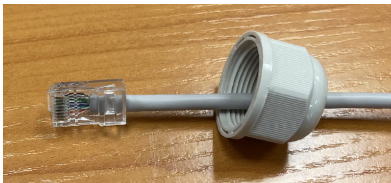
Рисунок 17 — Установка гайки кабельного ввода на кабеле
