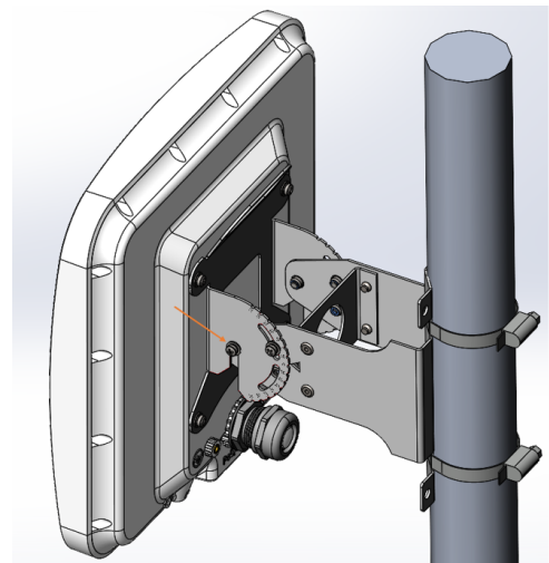
Рисунок 14 — Фиксация винтов
