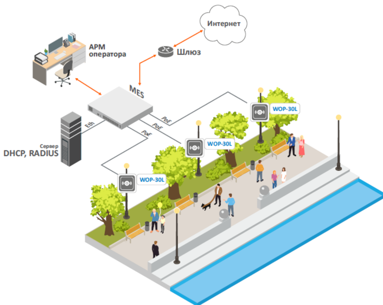
Рисунок 1 — Функциональная схема использования WOP-30L
