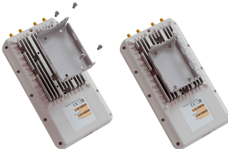
Рисунок 8 — Крепление кронштейна к устройству
