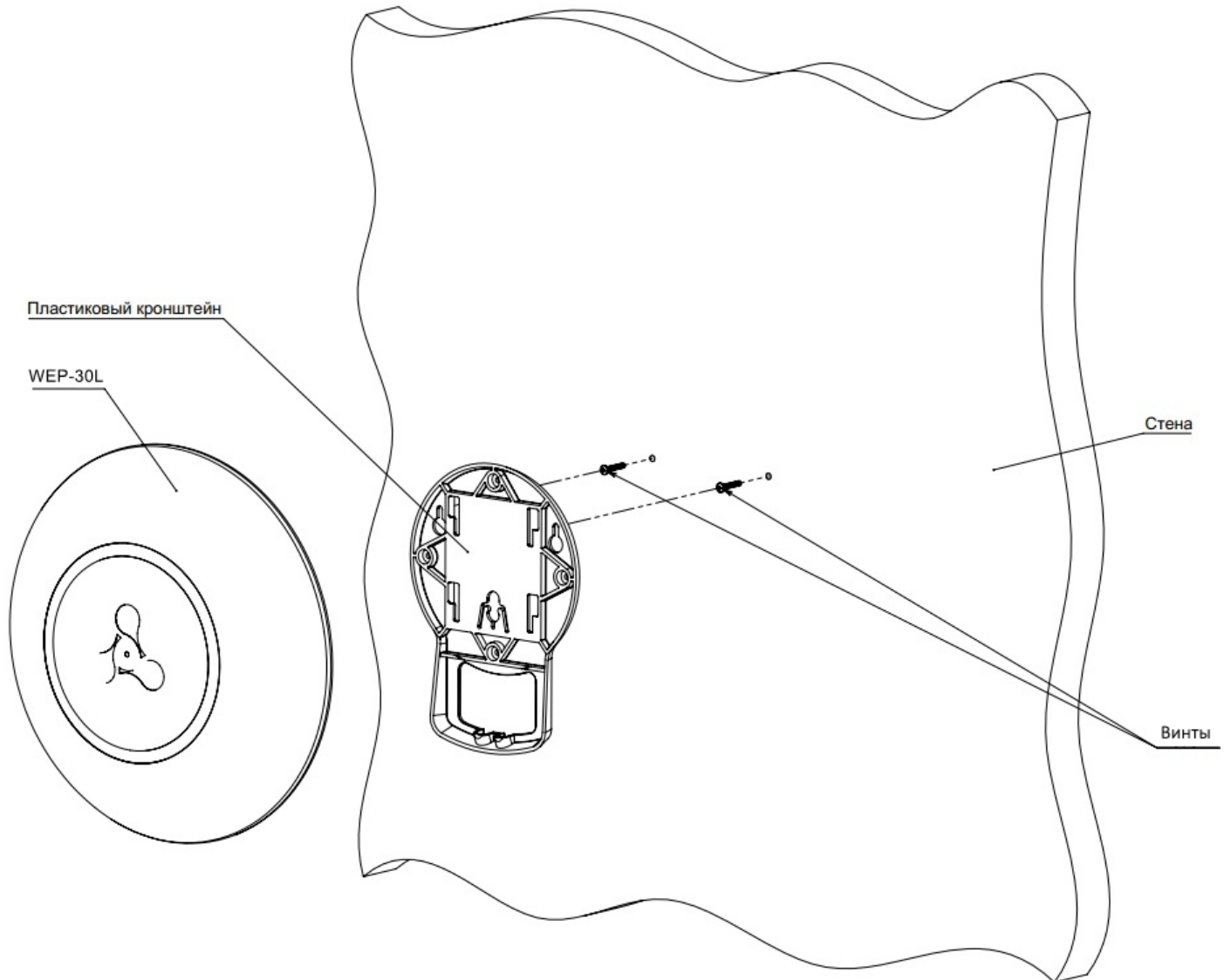
Рисунок 8 — Крепление кронштейна на стене
