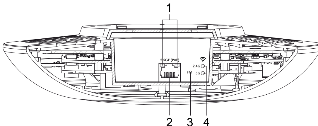
Рисунок 2 — Внешний вид основной панели WEP-30L
