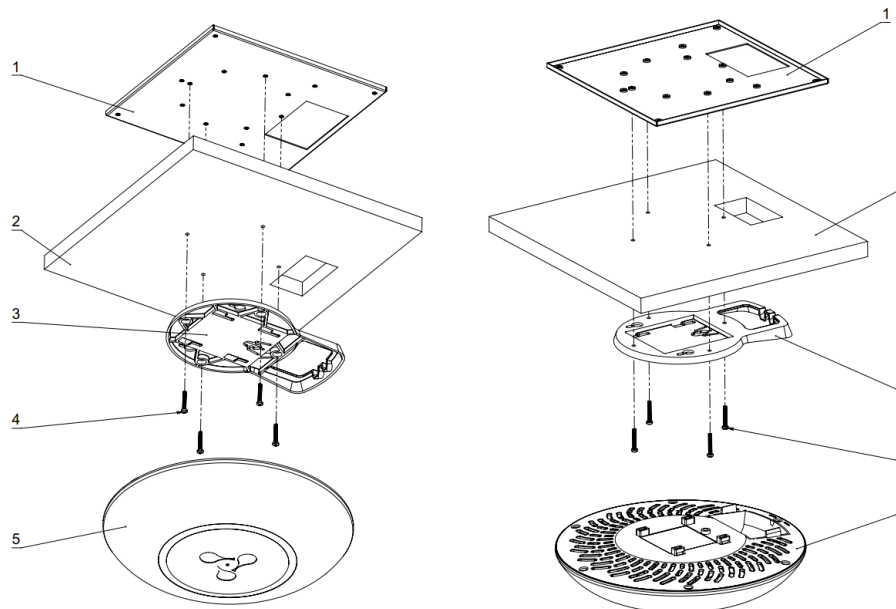
1 — металлический кронштейн; 2 — панель Армстронг; 3 — пластиковый кронштейн; 4 — винты; 5 — устройство.
