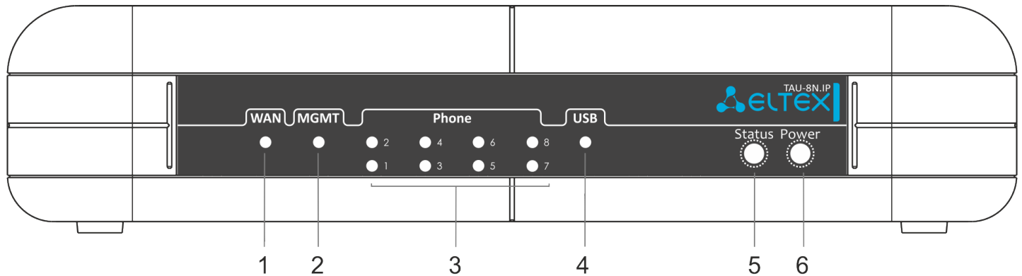
Рисунок 4 — Внешний вид передней панели TAU-8N.IP
