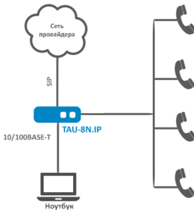
Рисунок 1 — Схема включения TAU-8N.IP
