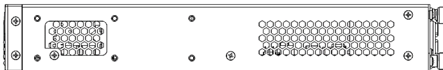
Рисунок 15 – Правая боковая панель Ethernet-коммутаторов MES5316A, MES5324A, MES5332A
