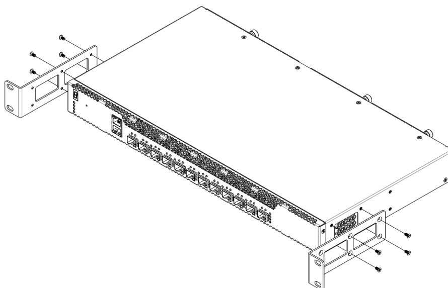
Рисунок 26 – Вариант крепления кронштейнов №2
