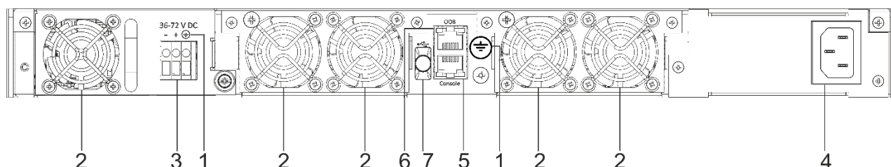
Рисунок 12 – Задняя панель MES5400-48
