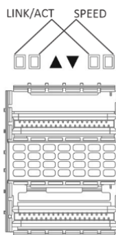
Рисунок 21 – Внешний вид разъема QSFP+
