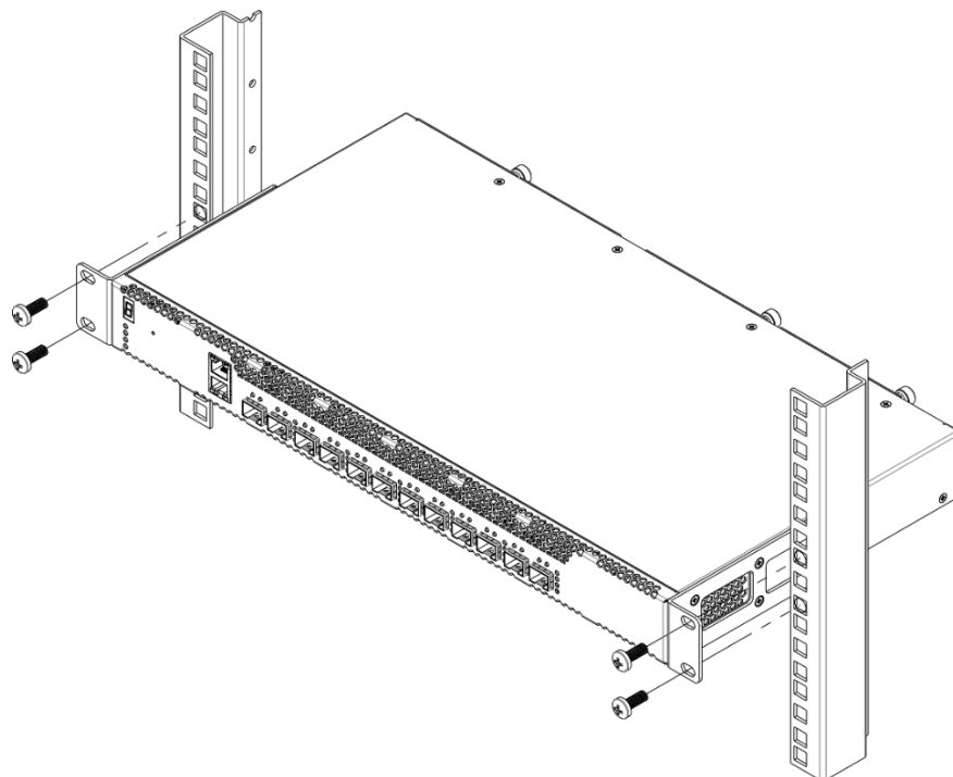
Рисунок 27 – Установка устройства в стойку
