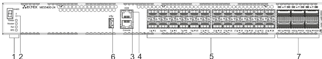
Рисунок 6 – Передняя панель MES5400-24
