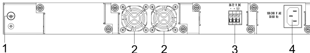
Рисунок 10 – Задняя панель MES5316A
