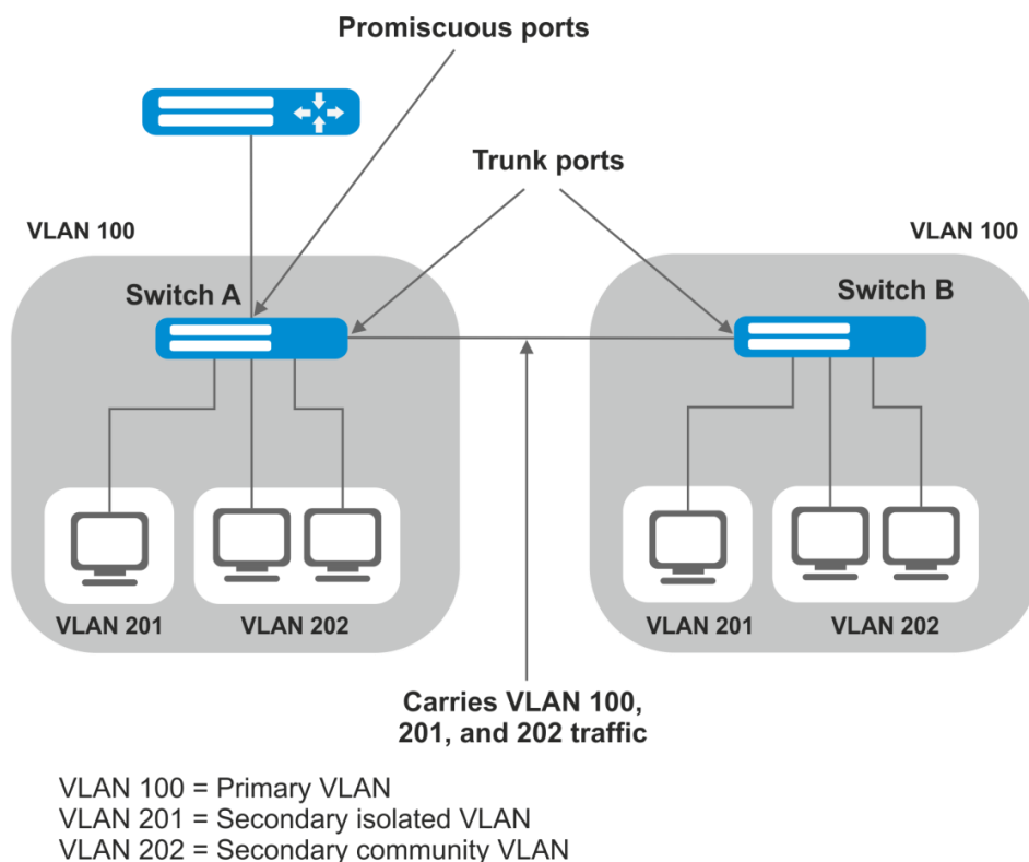
Рисунок 34 – Пример работы технологии Private VLAN
