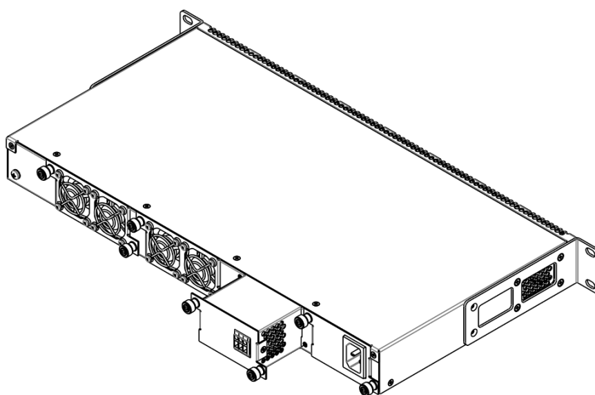
Рисунок 29 – Установка модулей питания
