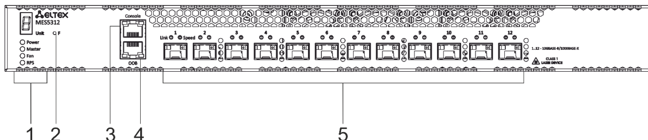
Рисунок 2 – Передняя панель MES5312
