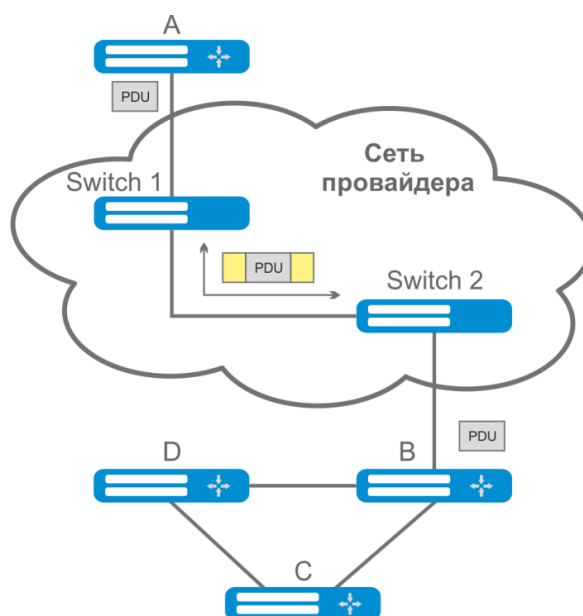
Рисунок 35 — Пример работы функции L2PT
