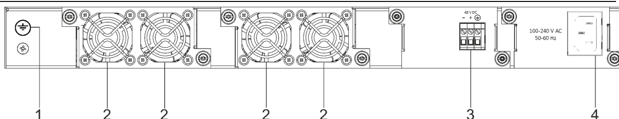
Рисунок 11 – Задняя панель MES5400-24
