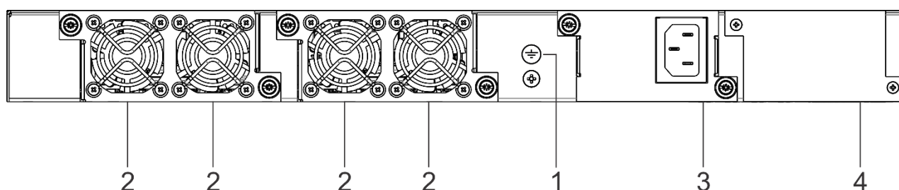
Рисунок 8 – Задняя панель MES3300-24F
