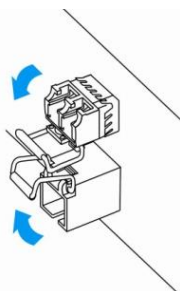
Рисунок 32 – Открытие защелки SFP-трансиверов
