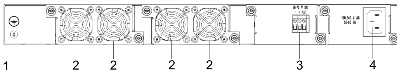
Рисунок 9 – Задняя панель MES5312, MES5324A, MES5332A
