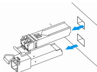
Рисунок 33 – Извлечение SFP-трансиверов
