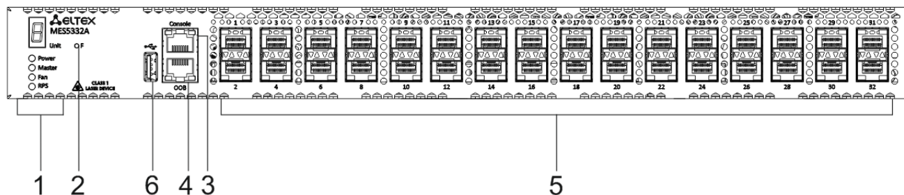
Рисунок 5 – Передняя панель MES5332A
