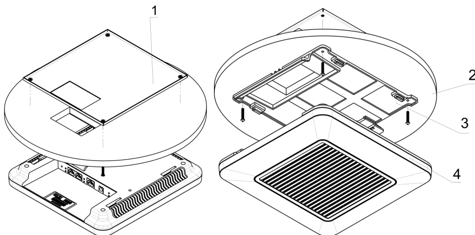
1 – металлический кронштейн; 2 – панель армстронг; 3 – пластиковый кронштейн; 4 – устройство. Рисунок 9 – Монтаж устройства на фальшпотолок
