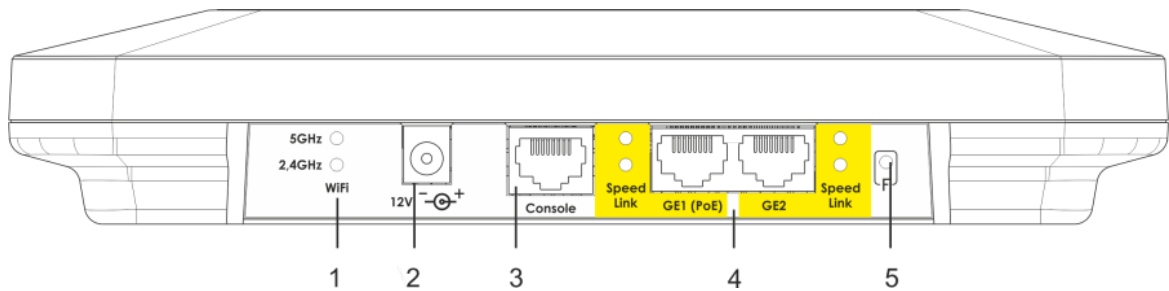
Рисунок 2 – Внешний вид основной панели WEP-12ac
