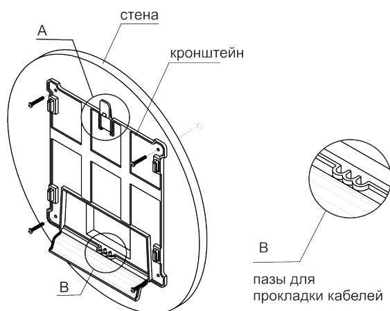
Рисунок 7 – Крепление кронштейна на стене
