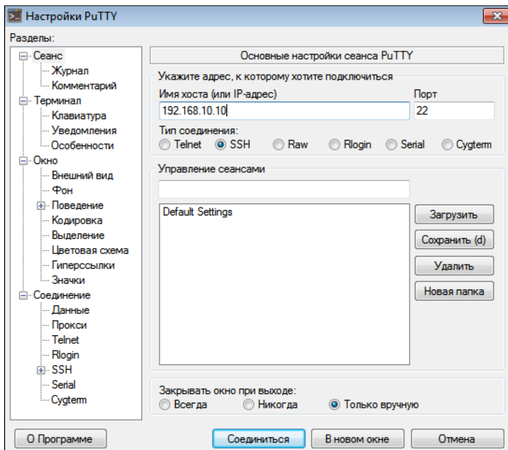
Рисунок 11 – Запуск SSH-клиента
