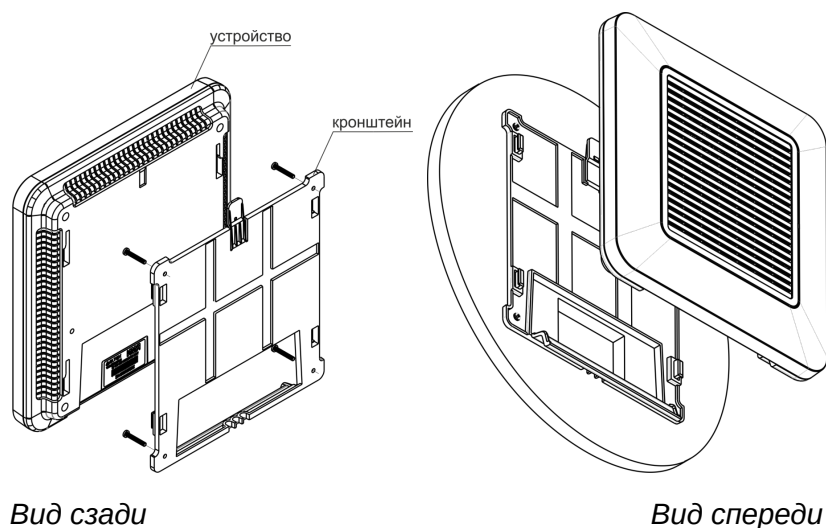
Рисунок 3 – Установка устройства
