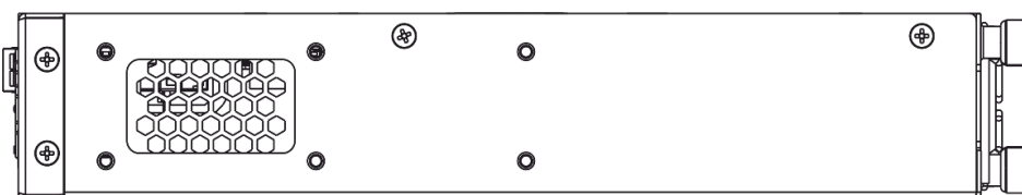
Рисунок 14 – Правая боковая панель Ethernet-коммутатора MES5312
